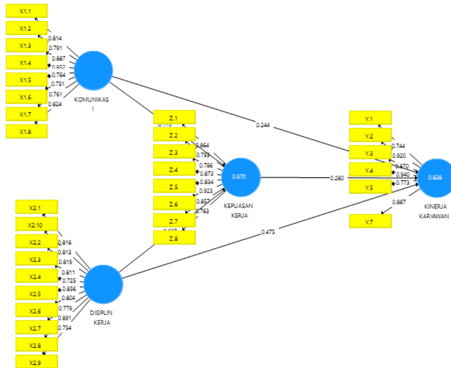
Gambar 2. Hasil Pengujian Outer Model
